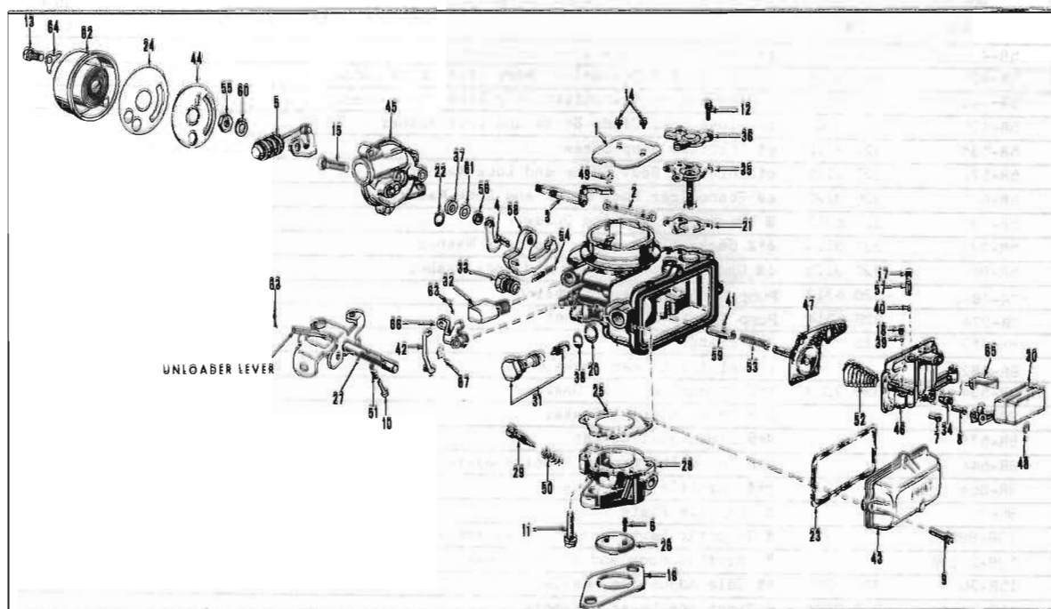
CARBURETOR 61 01 (OHV)
